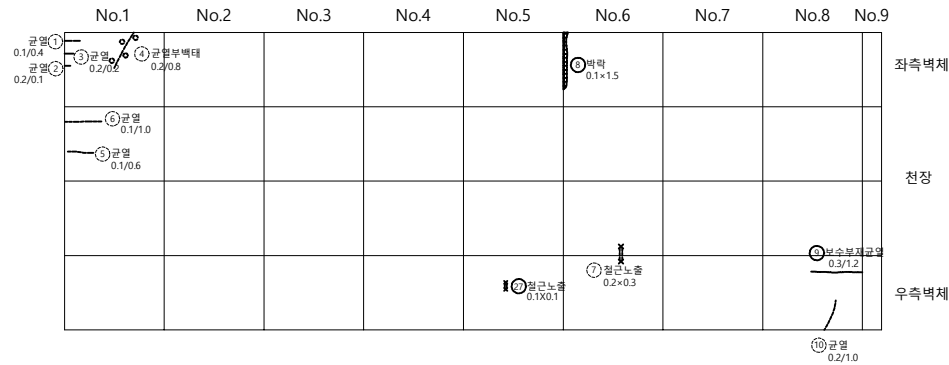
40 SPAN 피난연락통로
